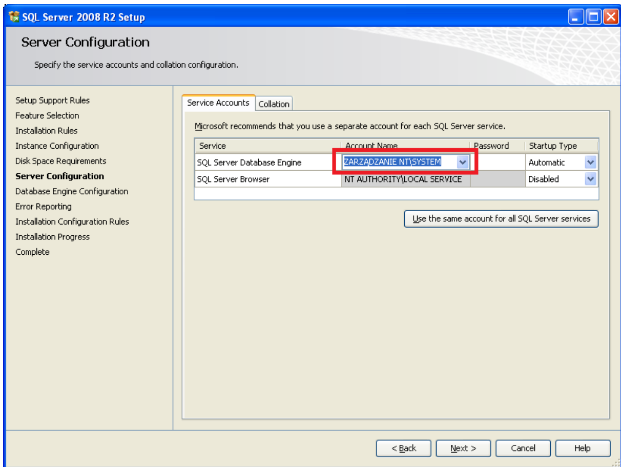
Rysunek 9: Konfiguracja serwera.
