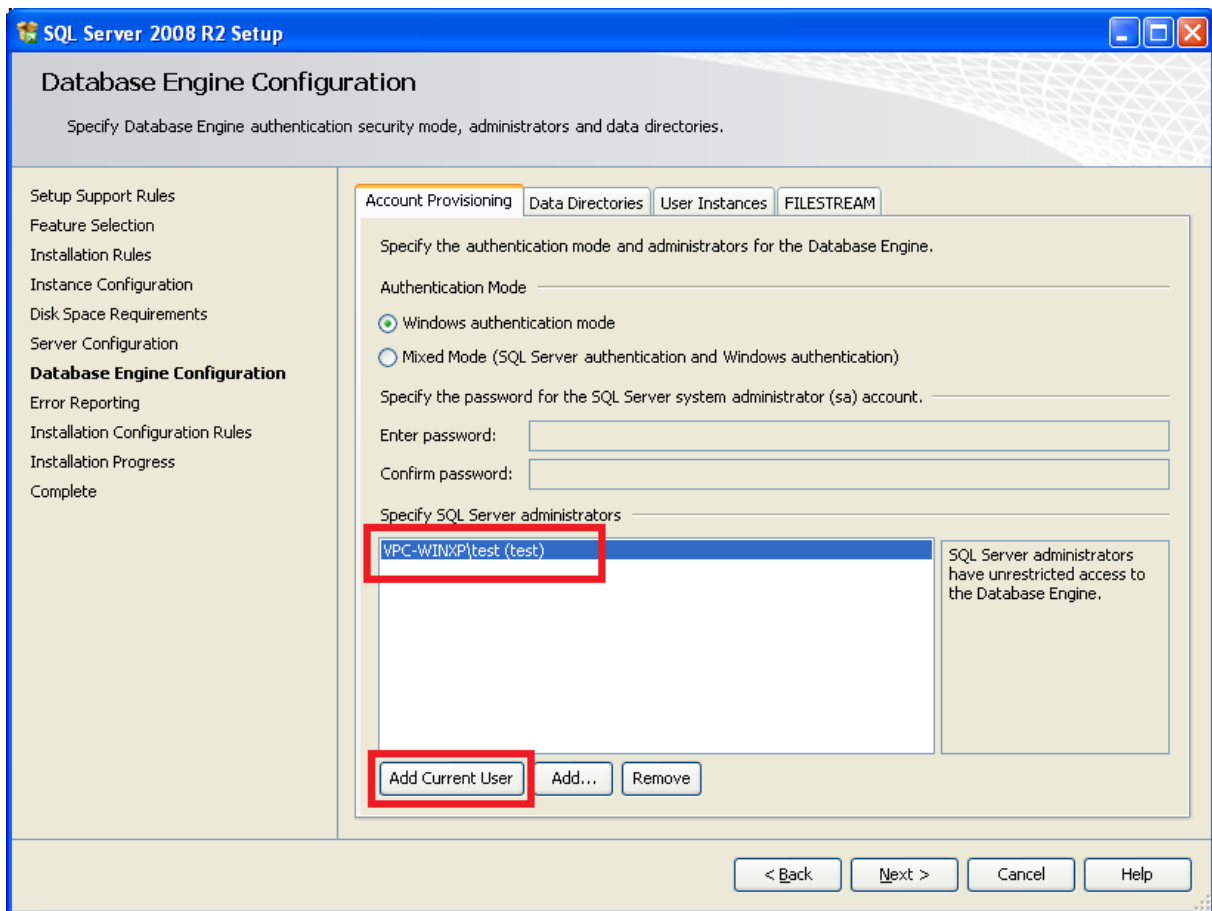
Rysunek 10: Konfiguracja silnika bazy danych.
